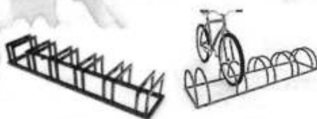
Suport pentru biciclete, 5 secții
